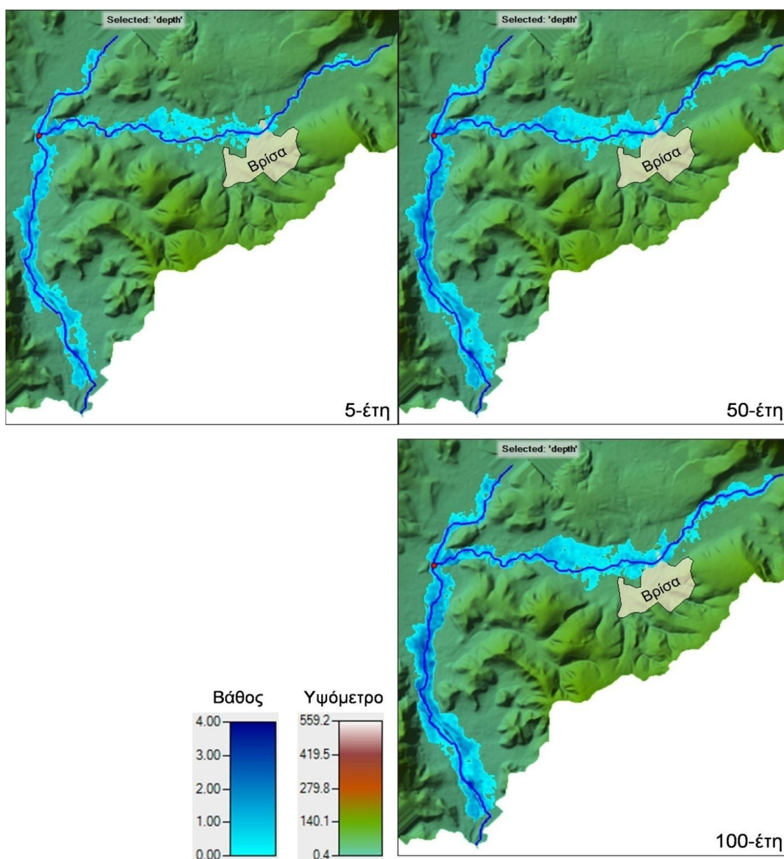
Εικόνα 3.2.2.19. Επιφάνεια κατάκλυσης και βάθος νερού κατά μήκος του υπό μελέτη τμήματος του ρ. Αλμυροπόταμου και για τις τρεις διαφορετικές περιόδους επαναφοράς (5, 50 και 100 έτη).
