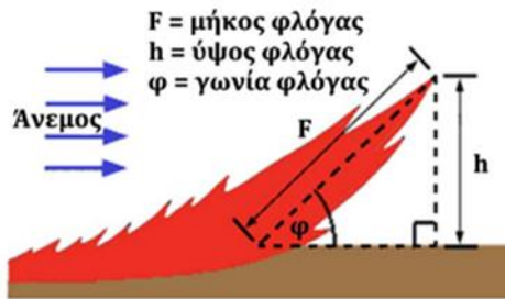
Εικόνα 3.1.1.27. Μήκος ( F ), ύψος ( h ) και γωνία φλόγας ( \varphi ) σε ένα δασικό πεδίο στο μέτωπο της πυρκαγιάς.
