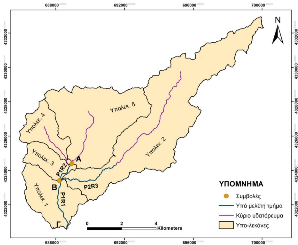
Εικόνα 3.2.2.13. Οι πέντε (5) υπο-λεκάνες στις οποίες υποδιαιρείται η λεκάνη απορροής του ρ. Αλμυροπόταμου, τα κύρια τμήματα του υδρογραφικού δικτύου με τα σημεία συμβολής αυτών (Α, Β), καθώς και οι κλάδοι του υδατορεύματος (P1R1, P1R2 και P2R3) που λαμβάνονται υπόψη κατά την υδραυλική προσομοίωση (υπό μελέτη τμήμα).
