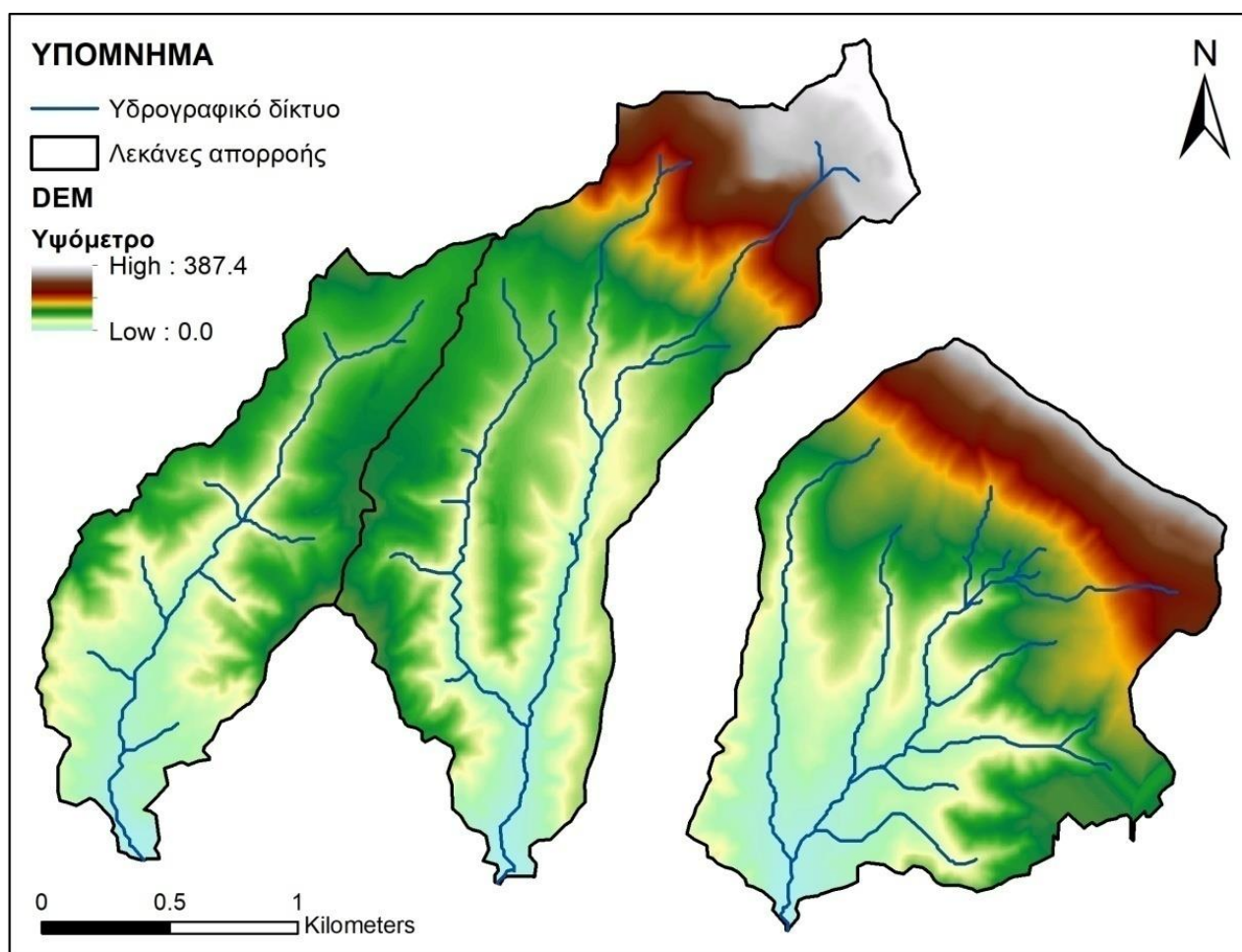
Εικόνα 3.2.2.9. Διαβάθμιση του εδαφικού αναγλύφου στις τρεις παρακείμενες λεκάνες απορροής.
