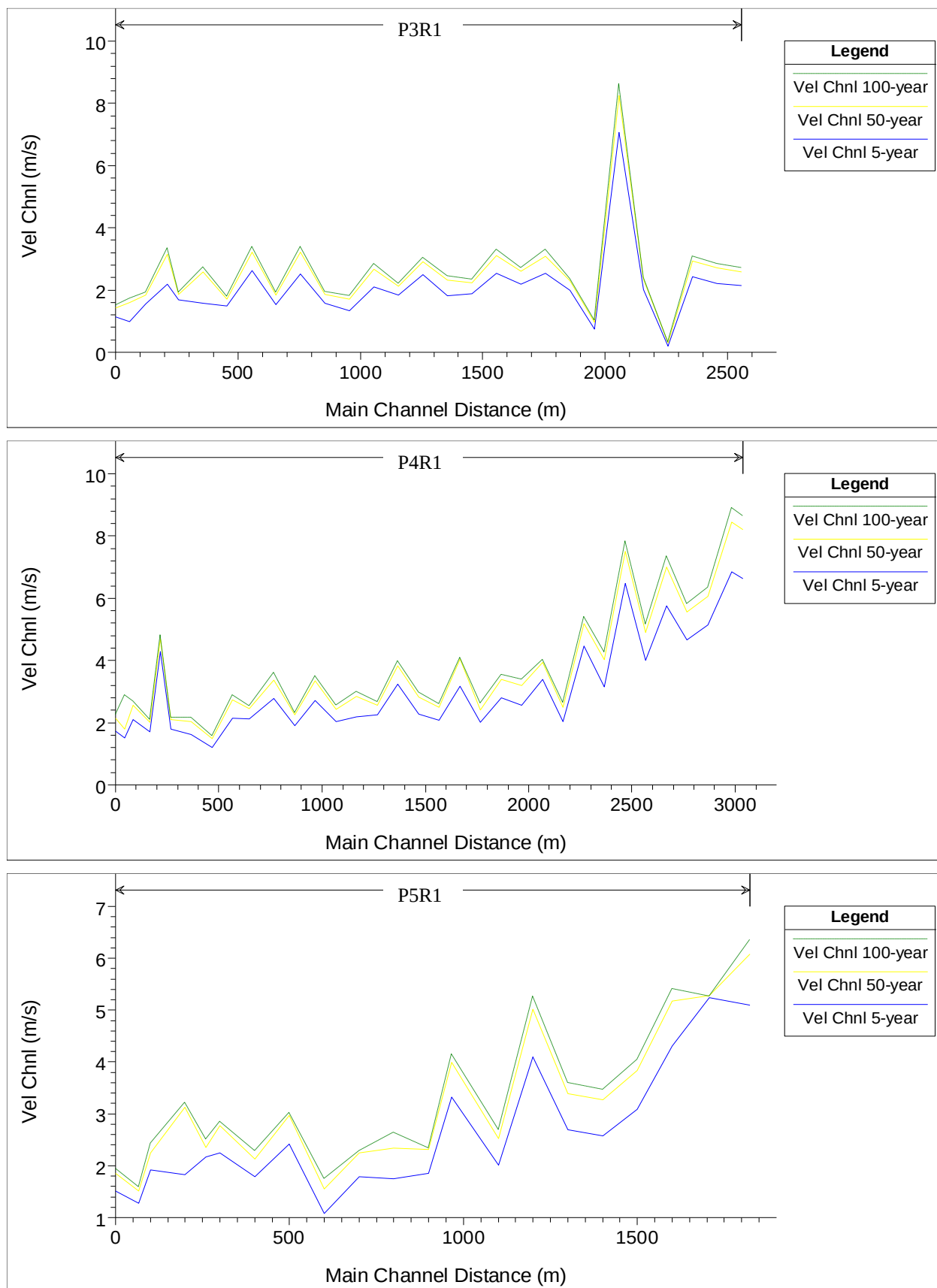
Εικόνα 3.2.2.18. Ταχύτητα ροής κατά μήκος των τριών υπό μελέτη κλάδων των παρακείμενων υδατορευμάτων (P3R1, P4R1 και P5R1) και για τις τρεις διαφορετικές περιόδους επαναφοράς (5, 50 και 100 έτη).
