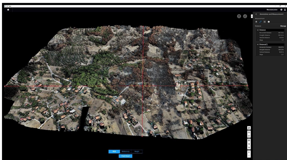
Εικόνα 3.7.2.15. 3d νέφος σημείων μέρους της περιοχής Βατερών – Διονύσου, με διαστάσεις 864 m x 566 m.
