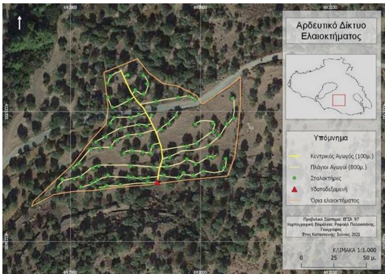
Εικόνα 3.3.16. Αρδευτικό δίκτυο ελαιοκτήματος.
