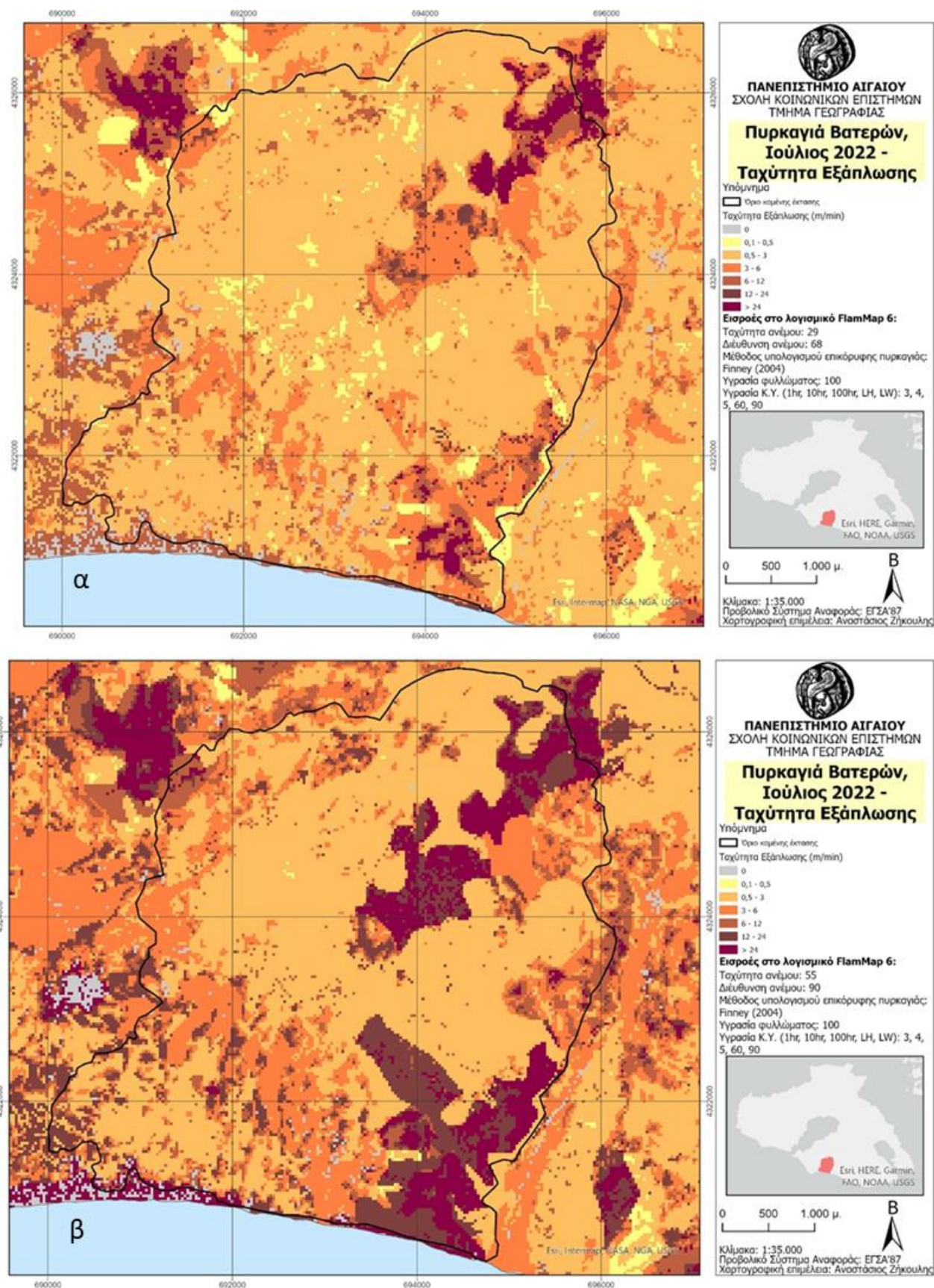
Εικόνα 3.1.1.33. Χάρτες ταχύτητας εξάπλωσης (m/min) πυρκαγιάς της περιοχής μελέτης με: (α) ταχύτητα ανέμου 5 Bf (29 km/h) και διεύθυνση ανέμου ABA (68°), και (β) ταχύτητα ριπής ανέμου 7 Bf (55 km/h) και διεύθυνση ανέμου A (90°).
