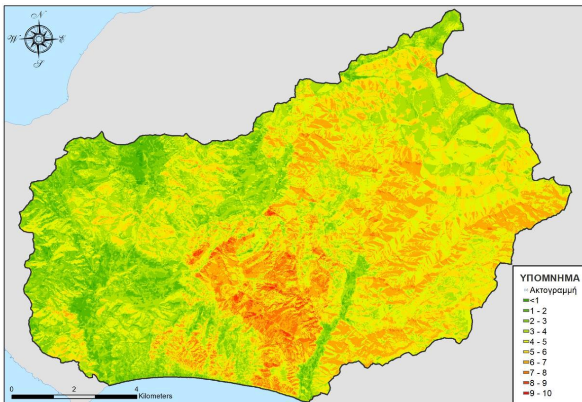
Χάρτης 3.2.1.11. Επικινδυνότητα διάβρωσης με βάση το 2ο Σενάριο.
