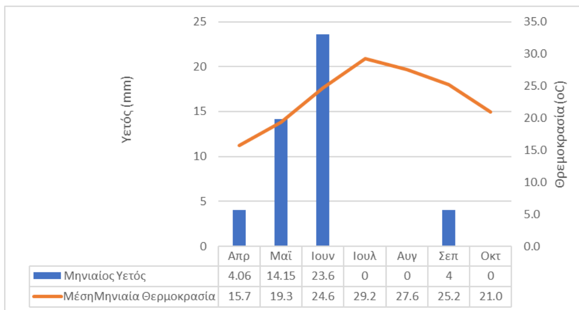
Εικόνα 4.7. Κατανομή μέσης μηνιαίας θερμοκρασίας (°C) και μηνιαίας βροχόπτωσης (mm), ΑΤΜΟΣ Βατερά, Απρίλιος-Οκτώβριος 2023.
